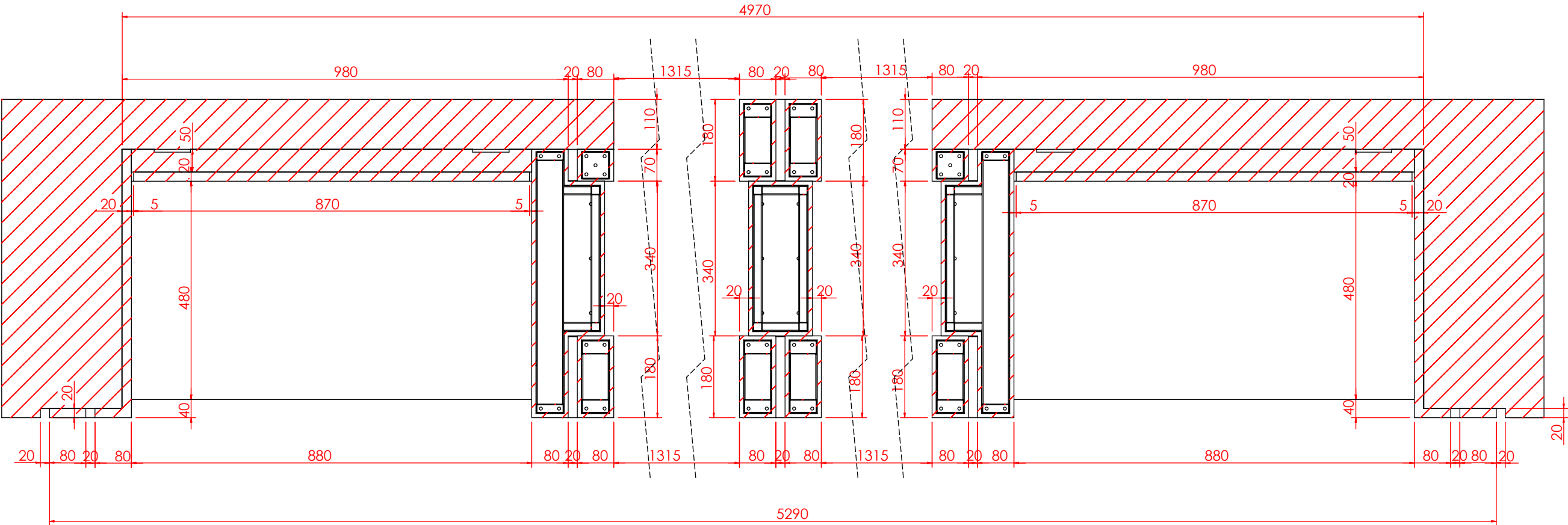
剖面 AI-AI
