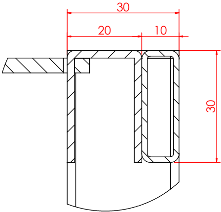
局部视图 B 比例 1 : 1
