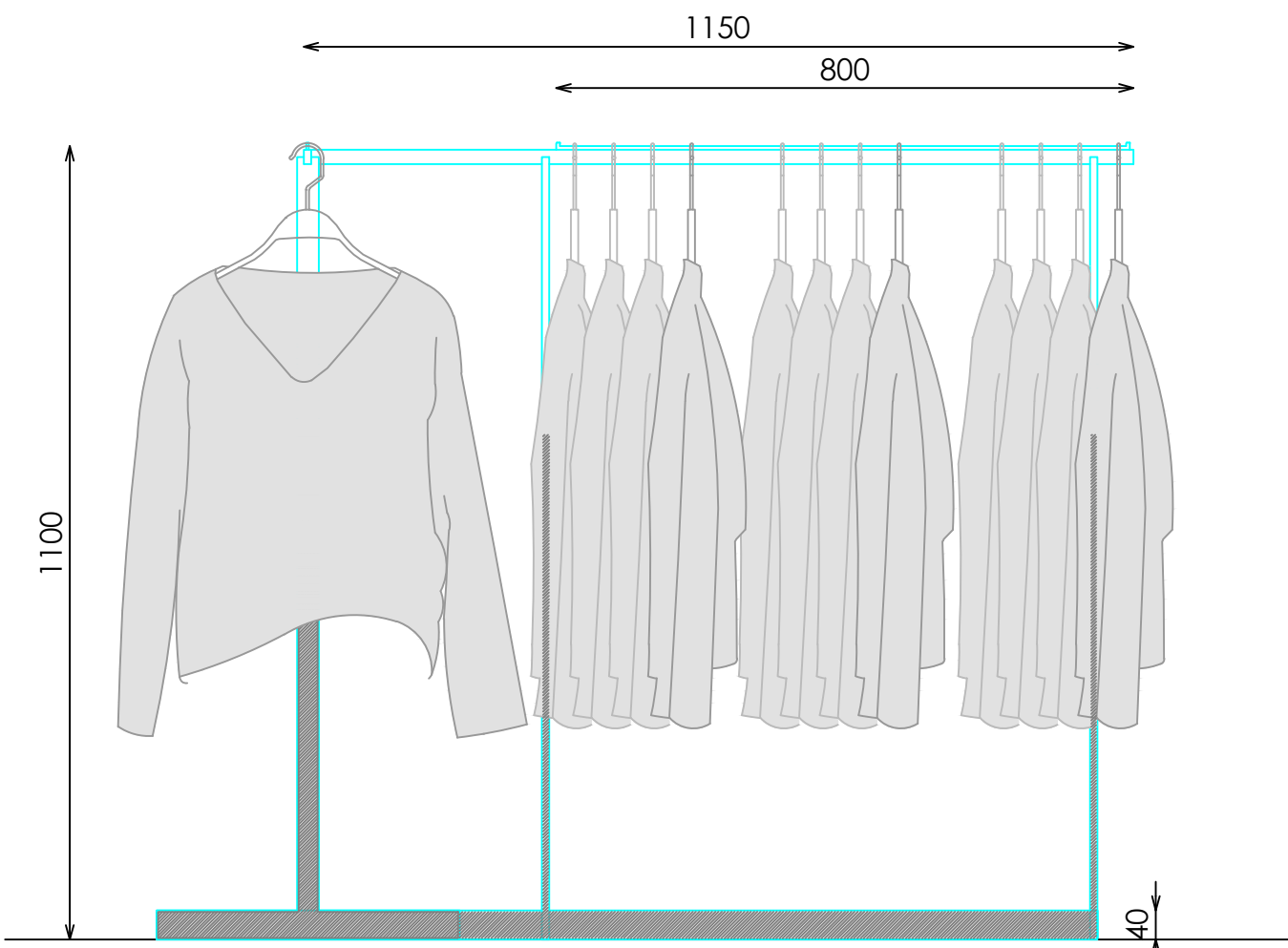
ALZADO FRONTAL
