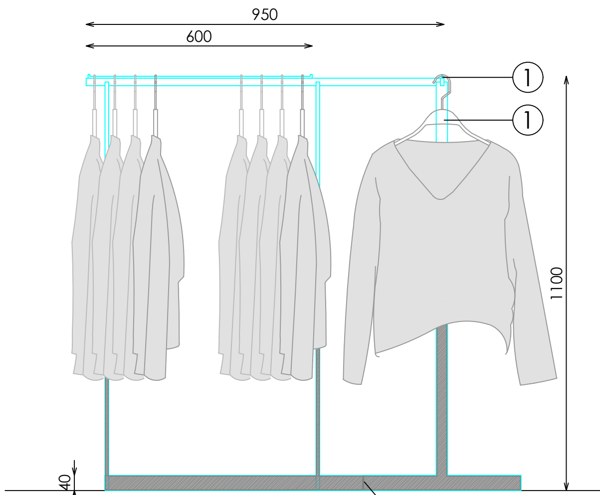
ALZADO LATERAL
