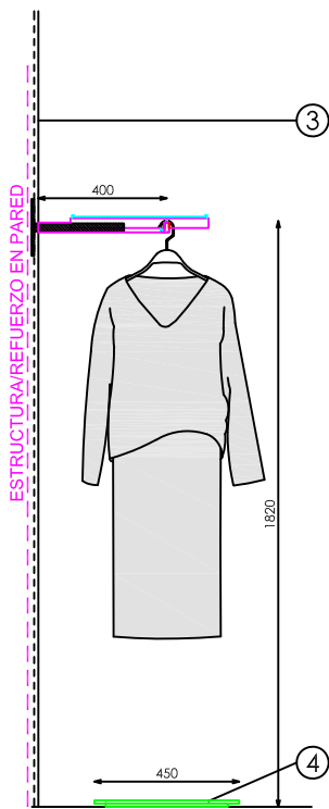
SECCIÓN BARRA
