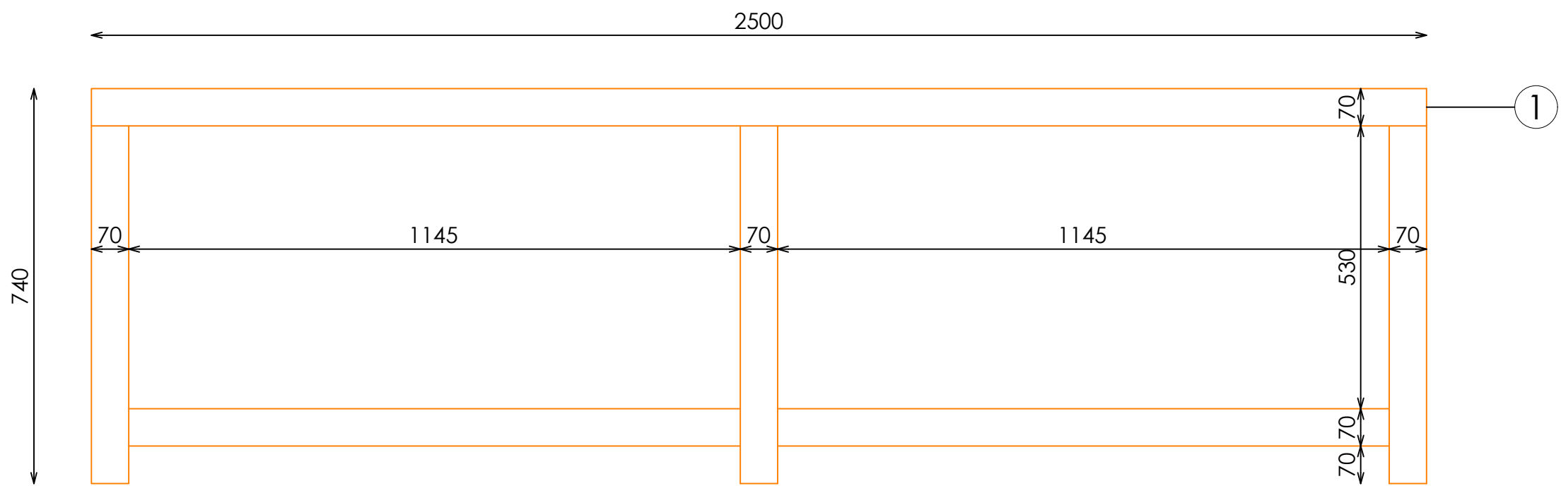
ALZADO FRONTAL
