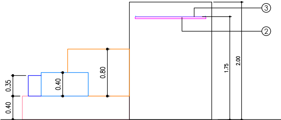
ALZADO POSTERIOR
