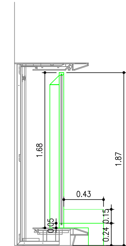
PERFIL
