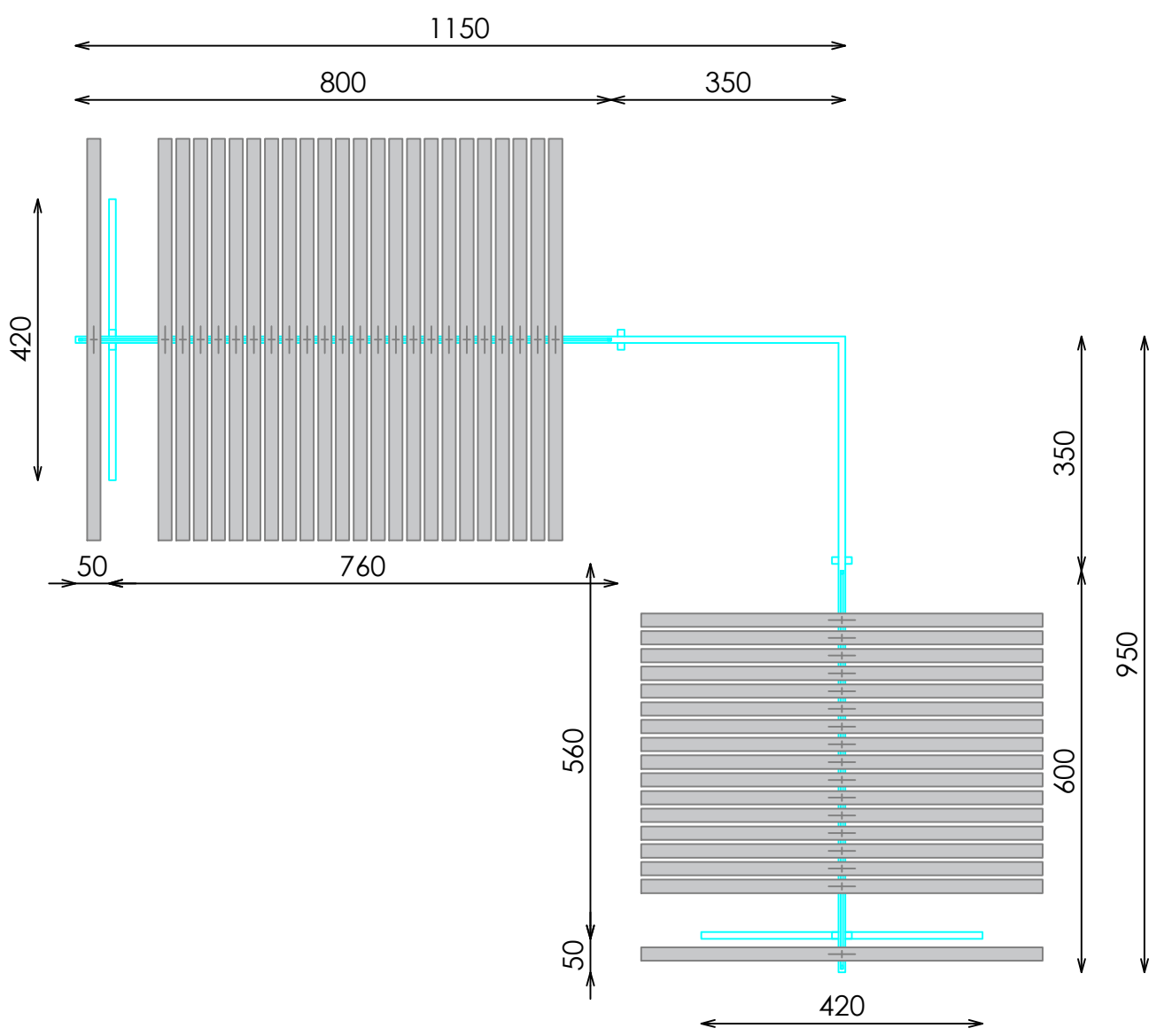
PLANTA
