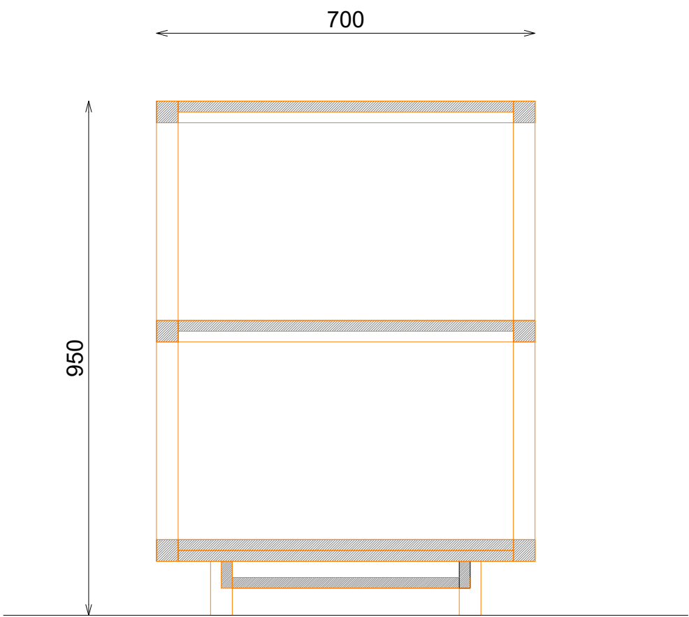
SECCION
