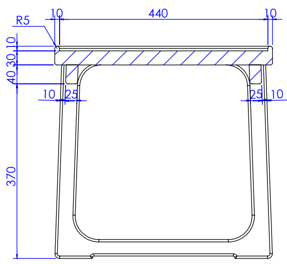
剖面 AJ-AJ
