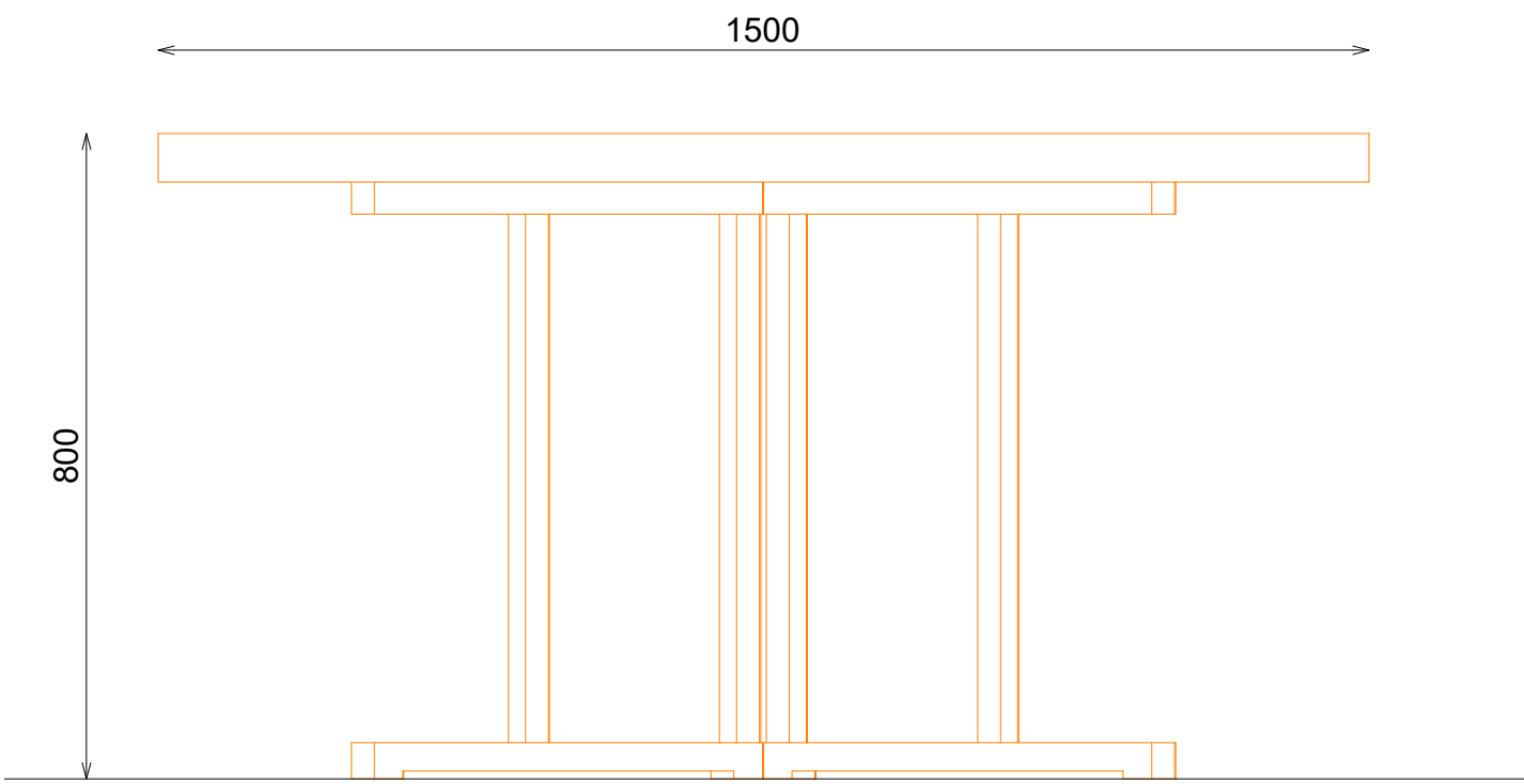
ALZADO LATERAL
