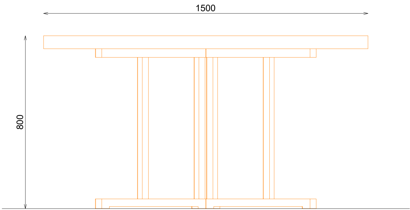
ALZADO FRONTAL
