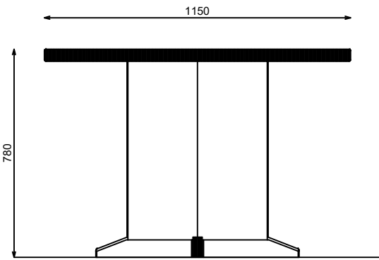
SECCION
