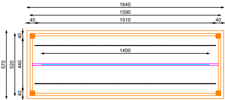
PLANTA
