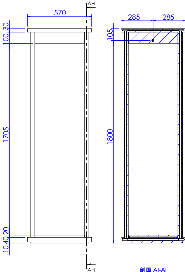
剖面 AI-AI
