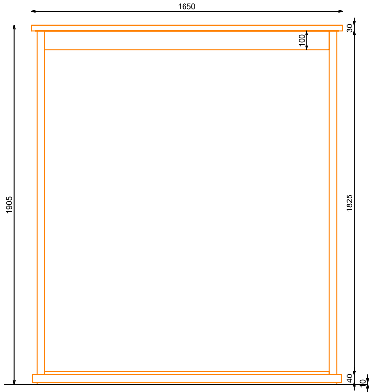
ALZADO
