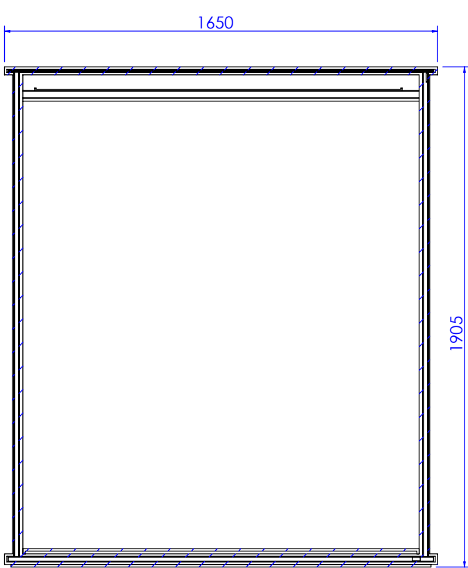
剖面 AH-AH
