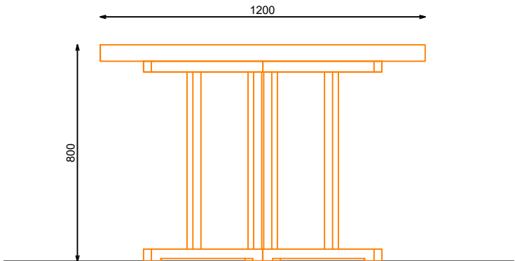
ALZADO LATERAL
