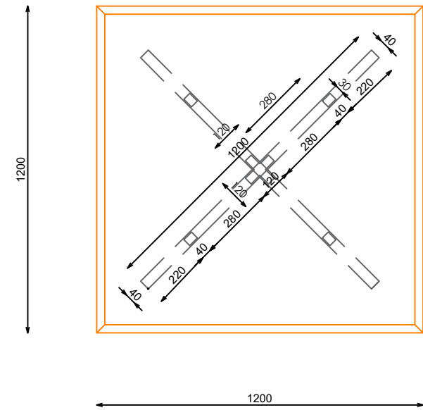
PLANTA
