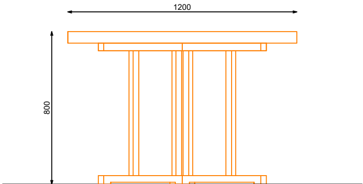
ALZADO FRONTAL
