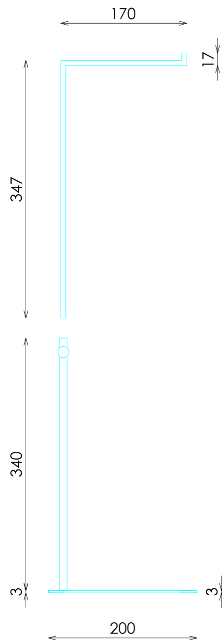
ALZADO
