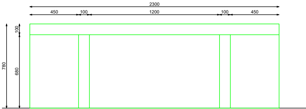
ALZADO FRONTAL
