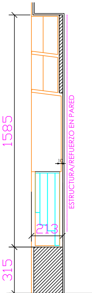
SECCION
