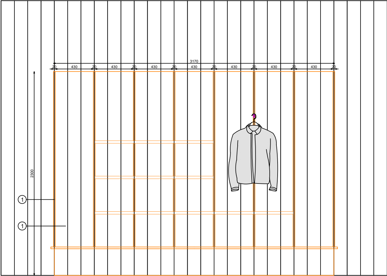
ALZADO FRONTAL
