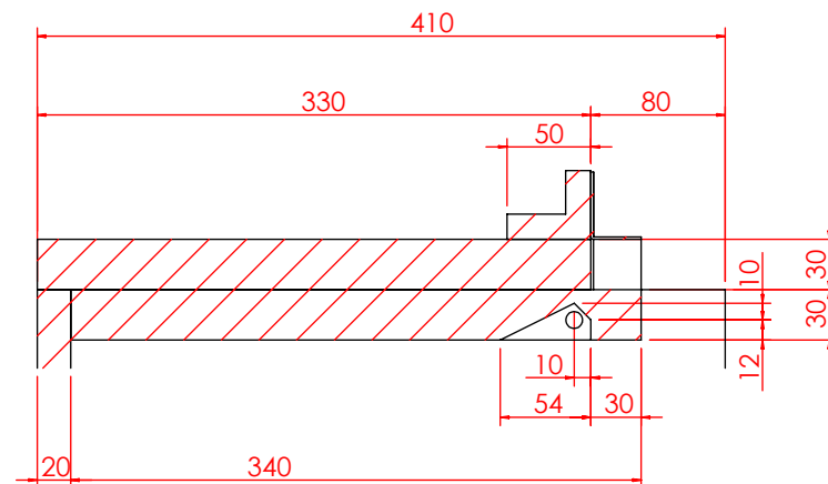
局部视图 AJ 比例 1 : 5
