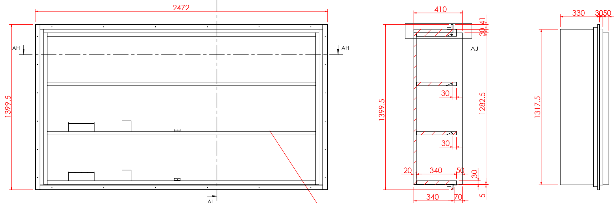
剖面 AI-AI
