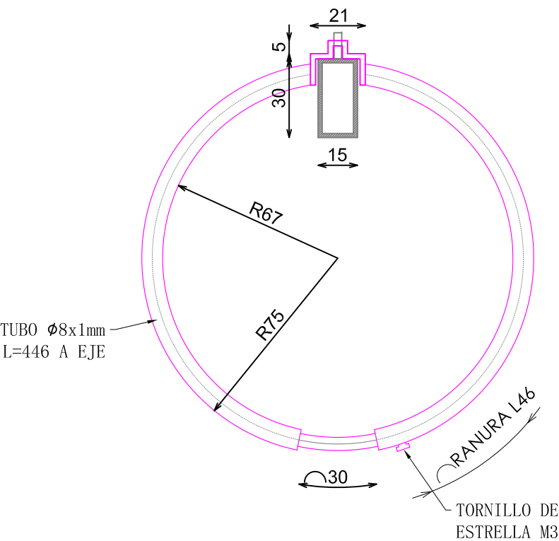
ALZADO
