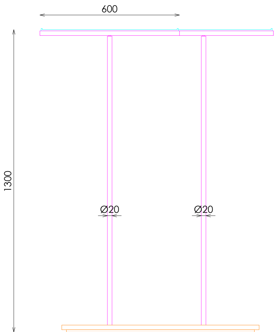
PERFIL IZQUIERDO
