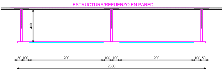
PLANTA
