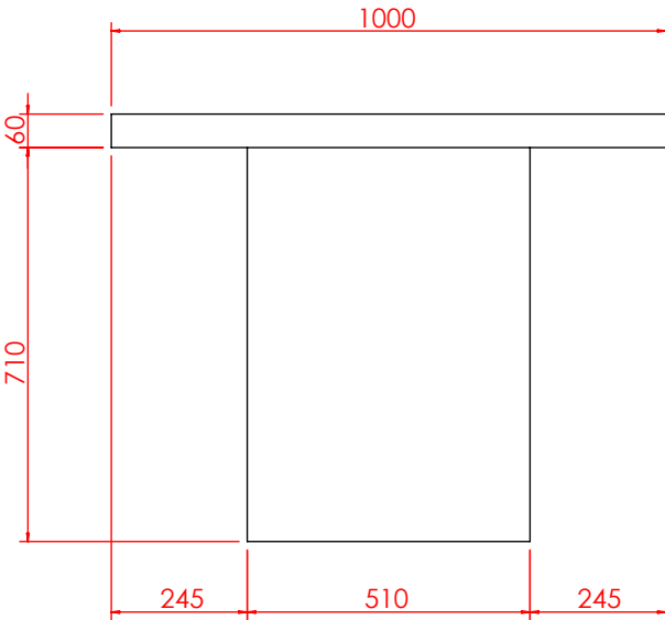
剖面 AK-AK
