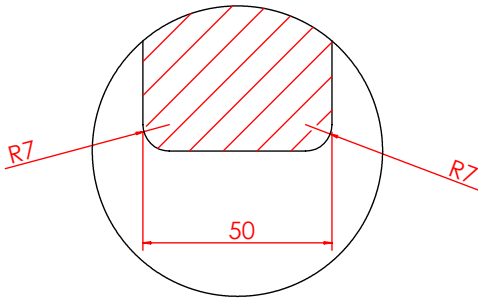
局部视图 AL 比例 1:2
