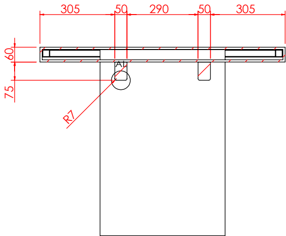
剖面 AK-AK
