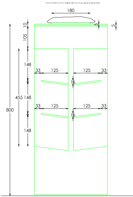
SECCION
