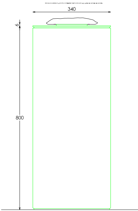
ALZADO LATERAL
