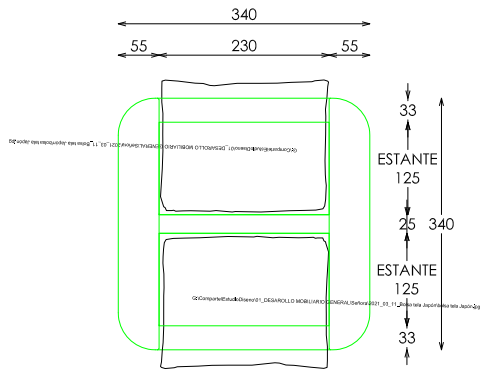
PLANTA SECCIONADA
