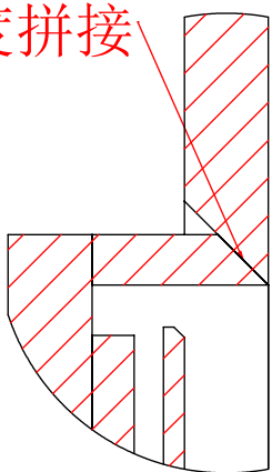
局部视图 AK 比例 1:2
