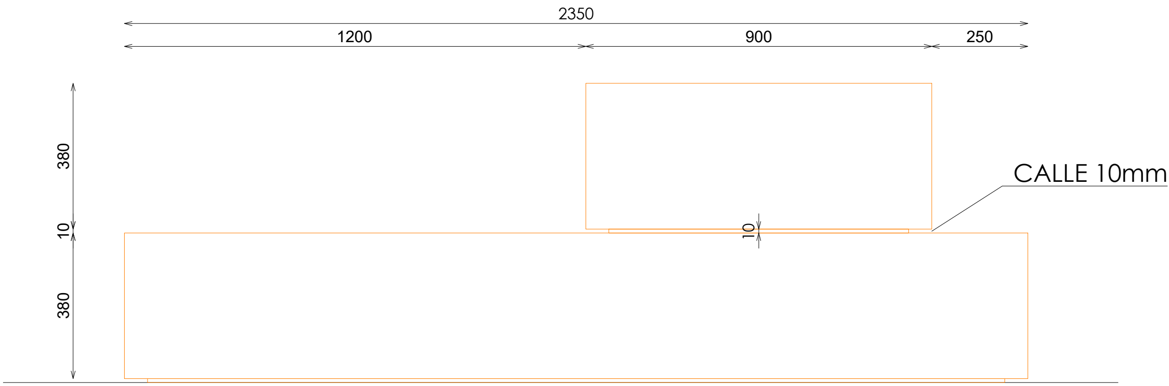
ALZADO LATERAL
