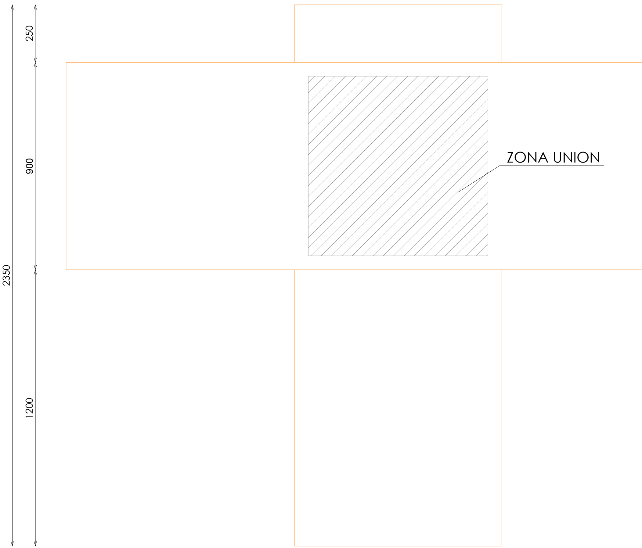
PLANTA
