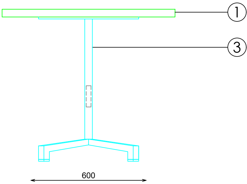
ALZADO LATERAL
