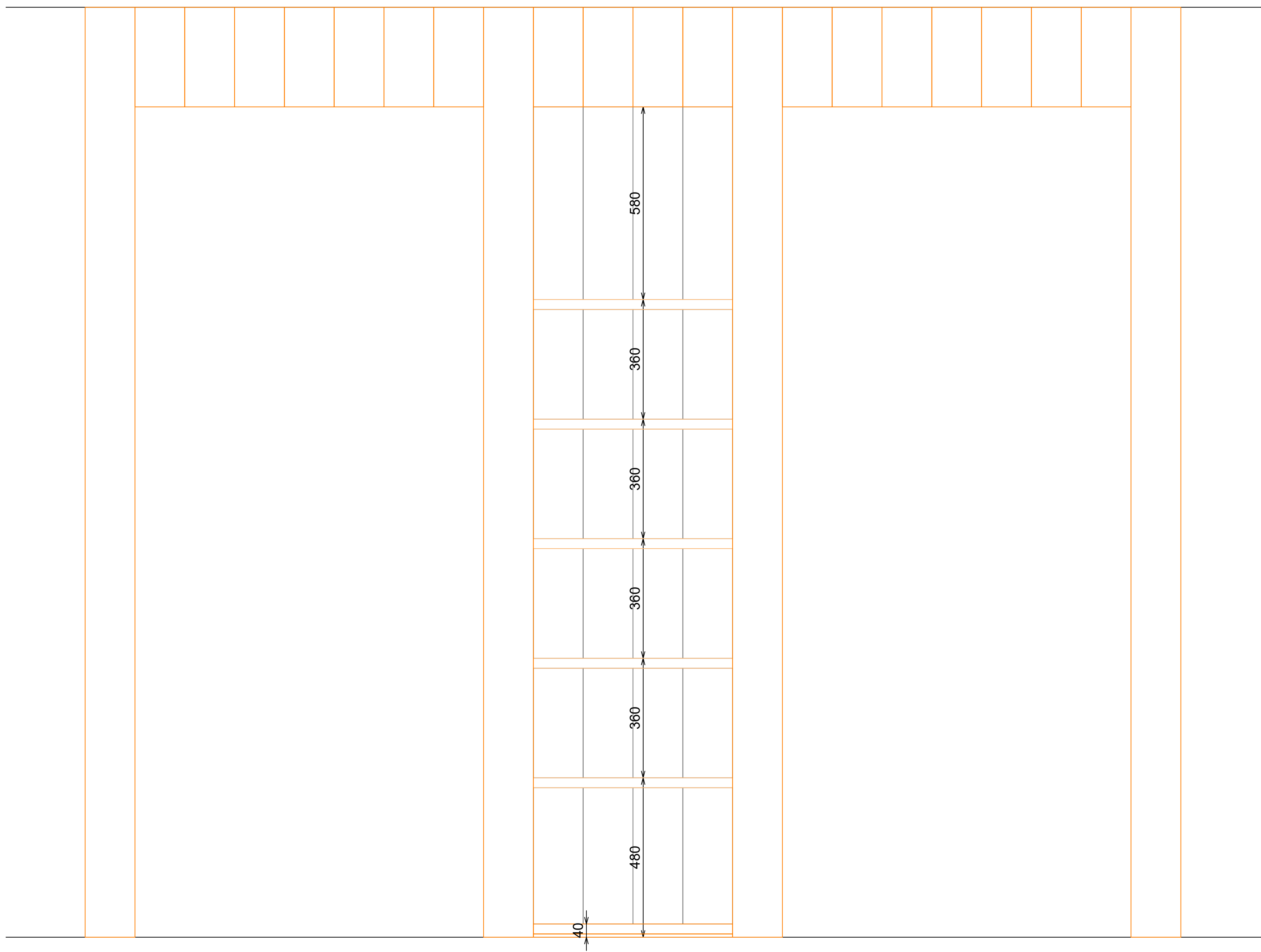
ALZADO
