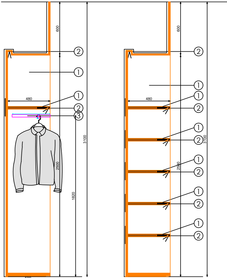
SECCION BARRA ALTA
