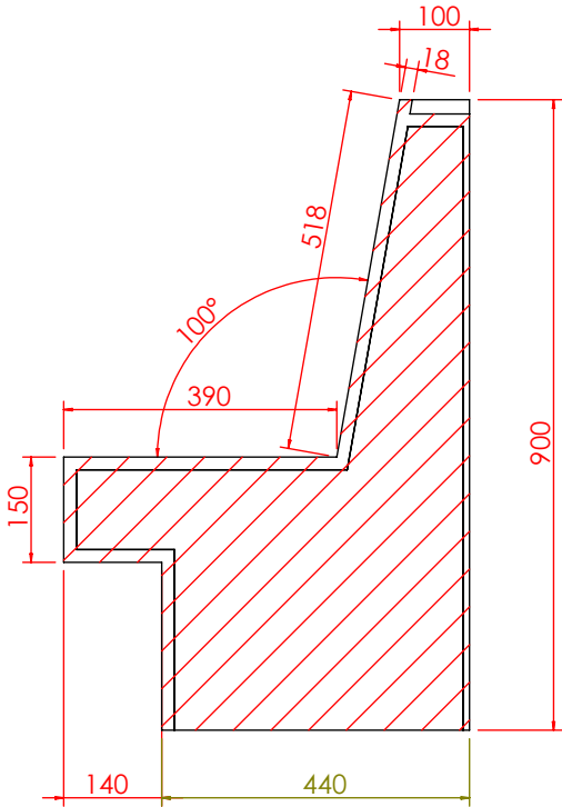
剖面 AL-AL 比例 1 : 12
