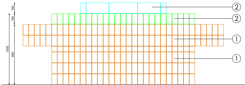
ALZADO LATERAL
