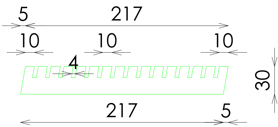
ALZADO
