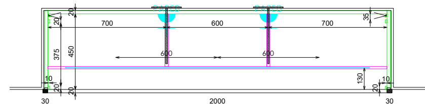
PLANTA B-B
