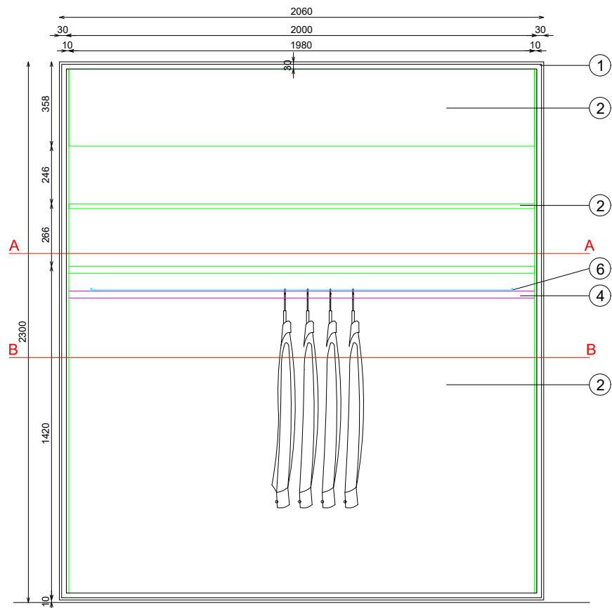
ALZADO FRONTAL
