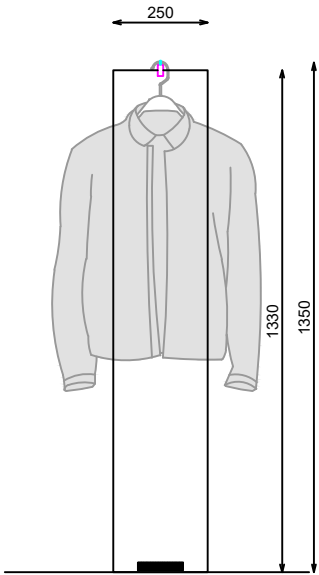
SECCION
