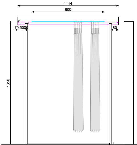
ALZADO
