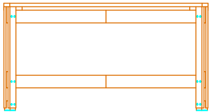
ALZADO LATERAL
