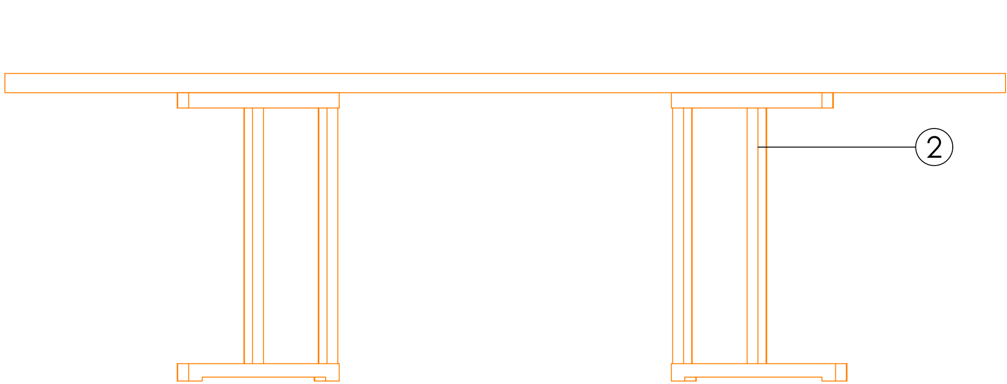
ALZADO FRONTAL
