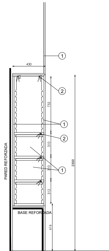
SECCIÓN
