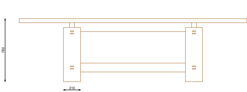
ALZADO FRONTAL
