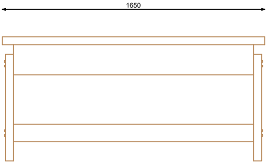
ALZADO LATERAL
