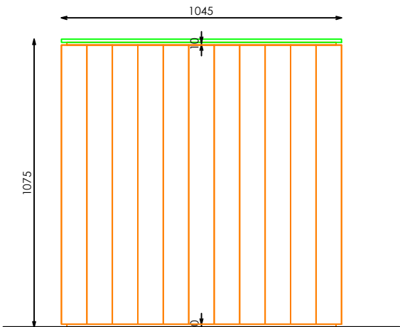
ALZADO FRONTAL
