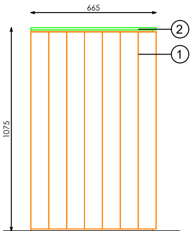
ALZADO LATERAL
