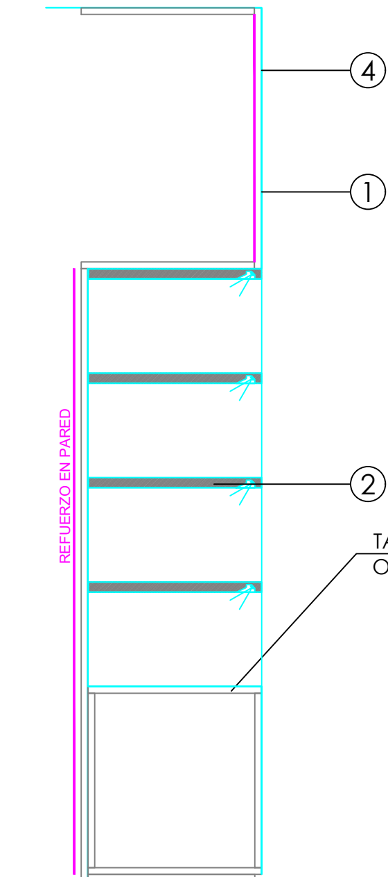
SECCIÓN BALDAS
