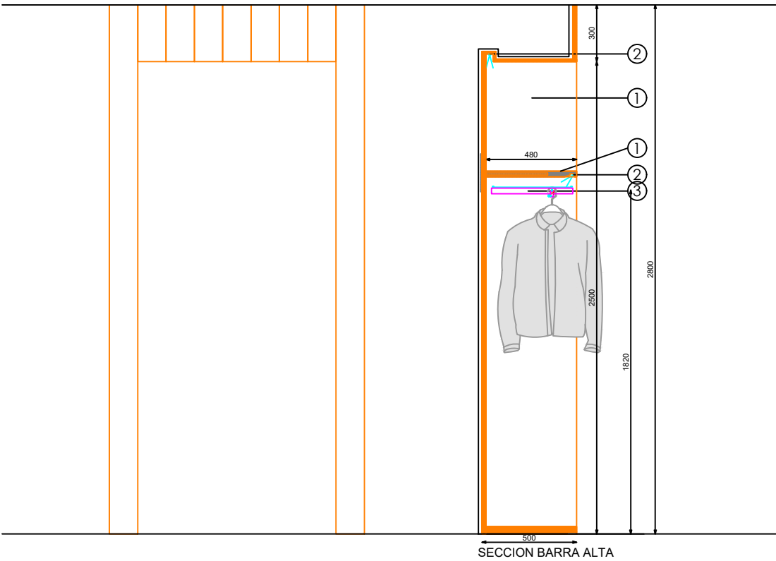
ALZADO
