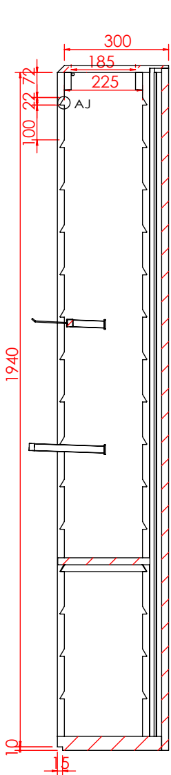
剖面 AI-AI 比例 1 : 15
