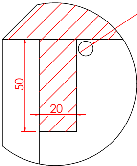
局部视图 AM 比例 1 : 2
