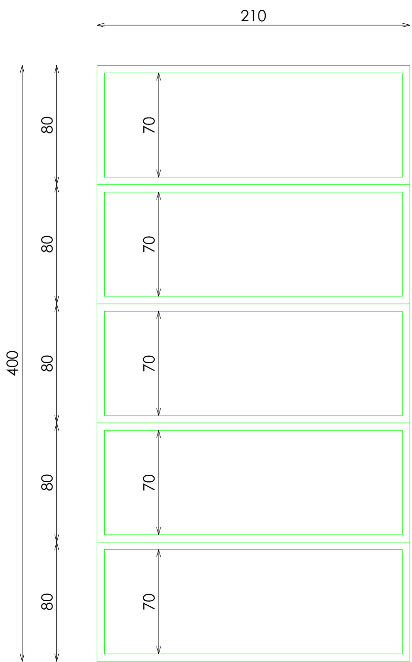
PLANTA
