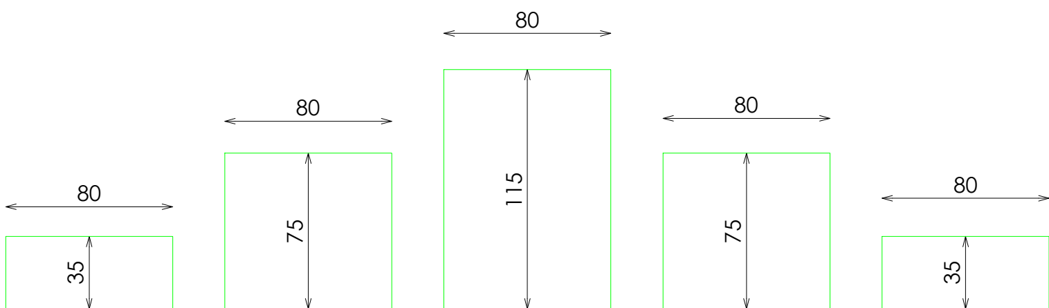
PERFIL
