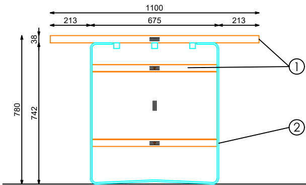
ALZADO LATERAL
