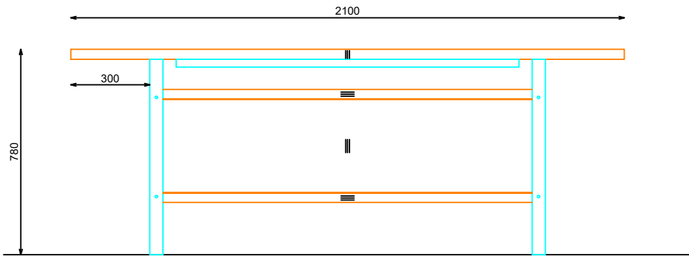
ALZADO FRONTAL
