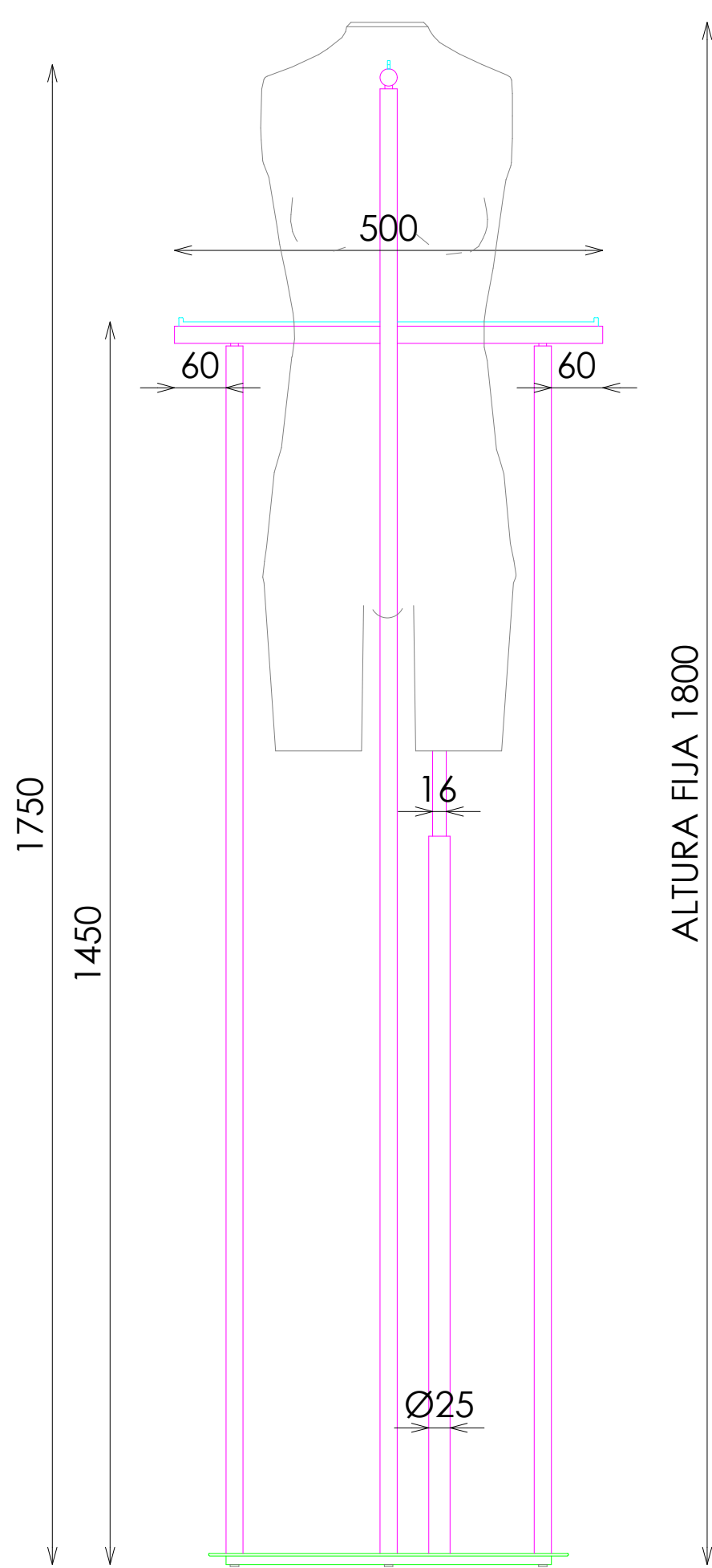
ALZADO FRONTAL
