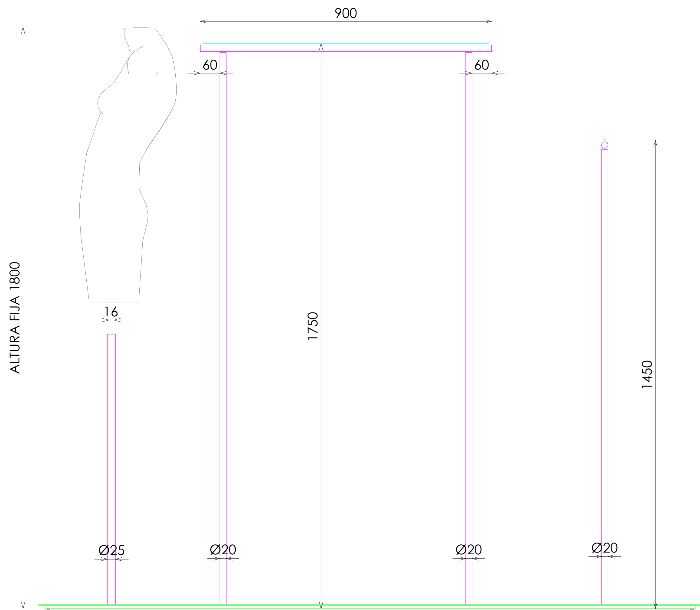
ALZADO LATERAL
