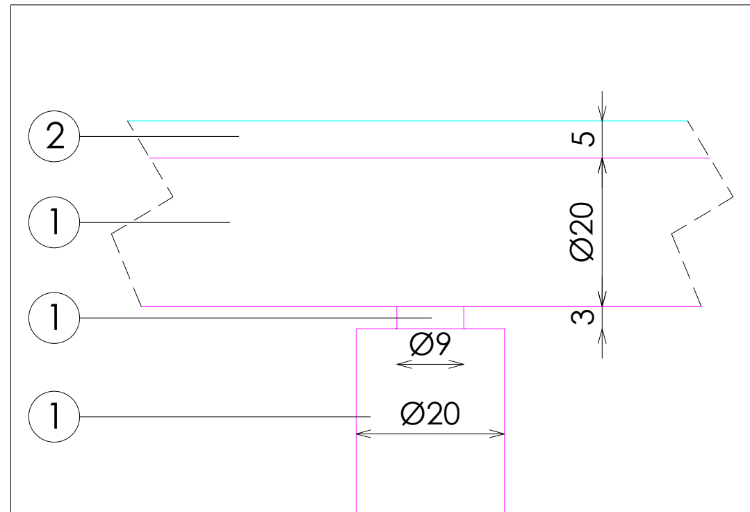
DETALLE B
