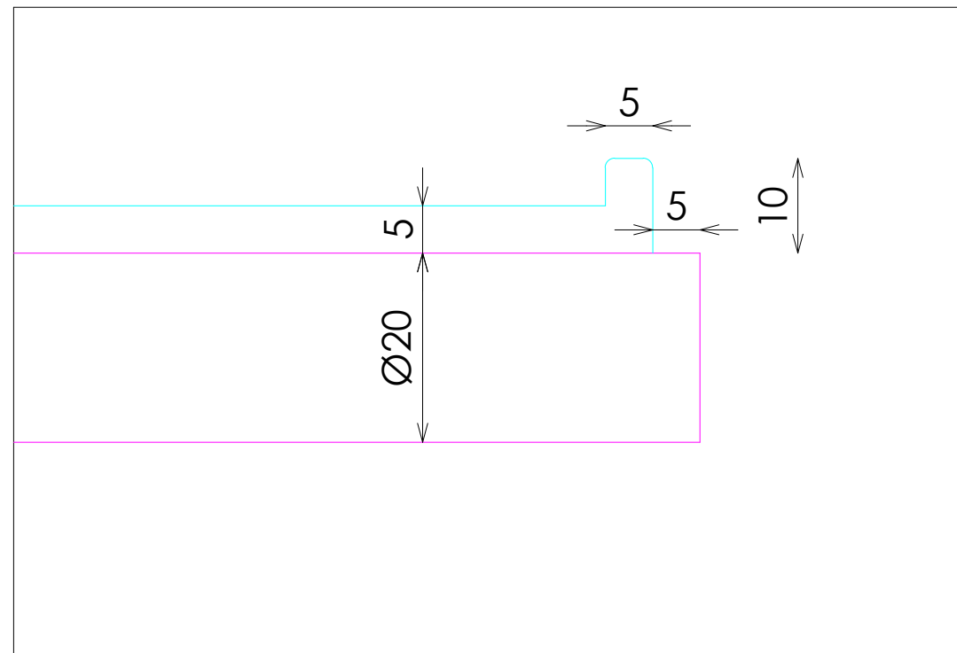
DETALLE C
