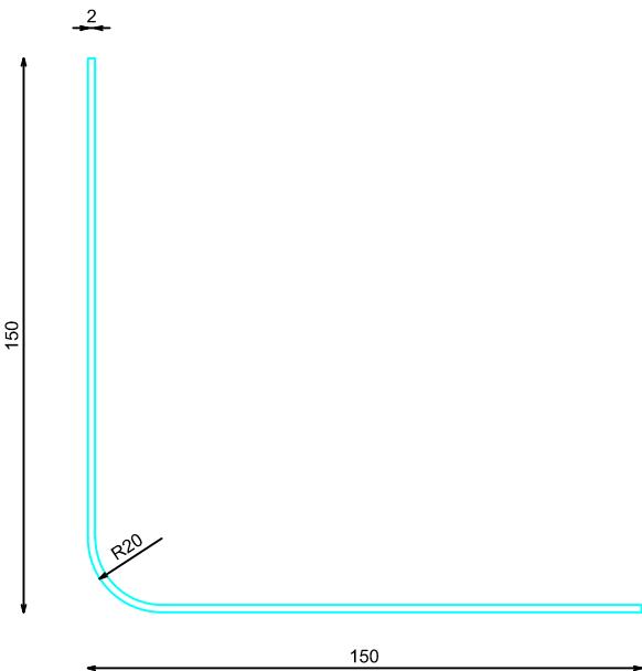
ALZADO
