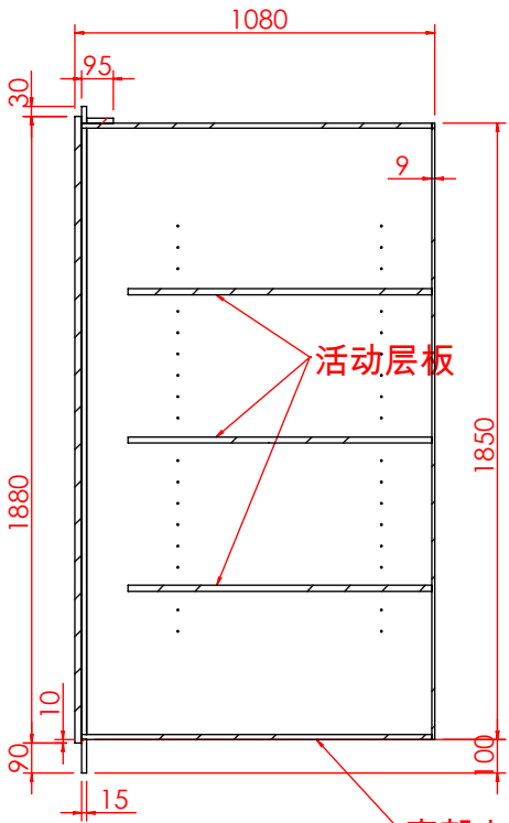
剖面 AG-AG 底部安装 黑色塑料调整脚
