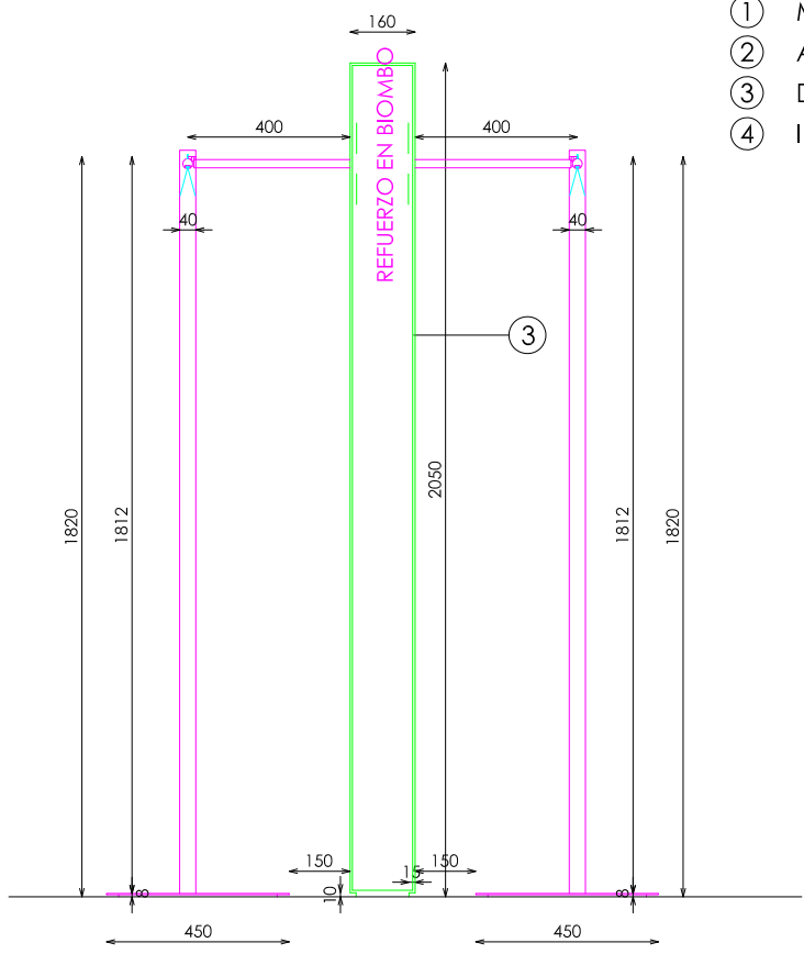
PERFIL
