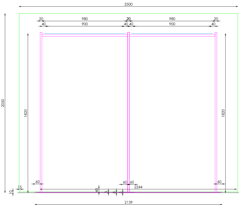
ALZADO
