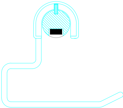
DETALLE MONTAJE BARRA Ø25
