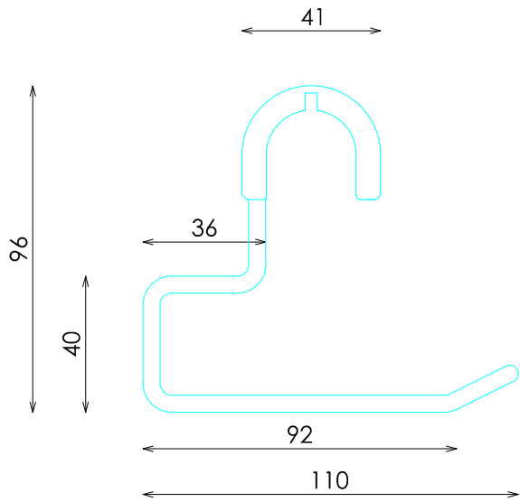
ALZADO
