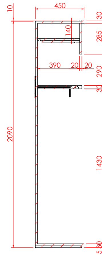
剖面 AH-AH
